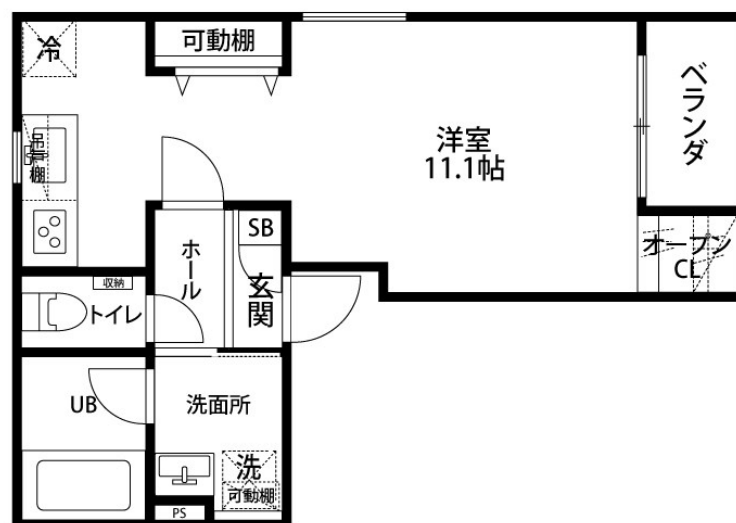
【間取り図】
