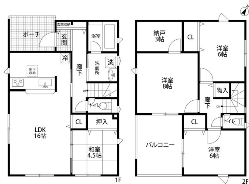
【間取り図】
